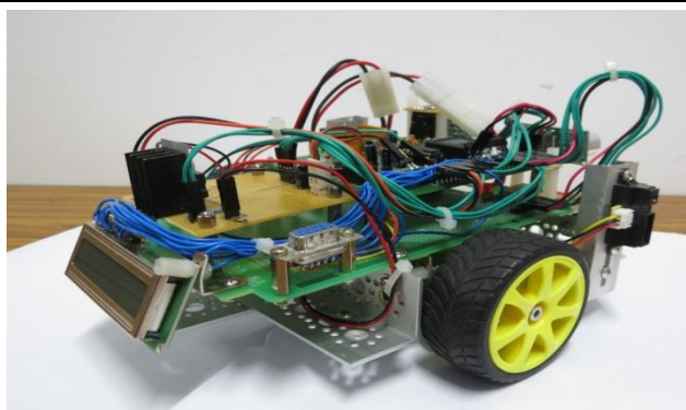
自走車正面
