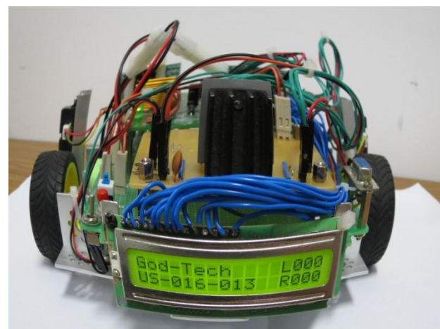
自走車正面特寫
