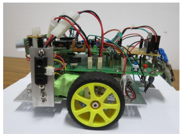
自走車側面
