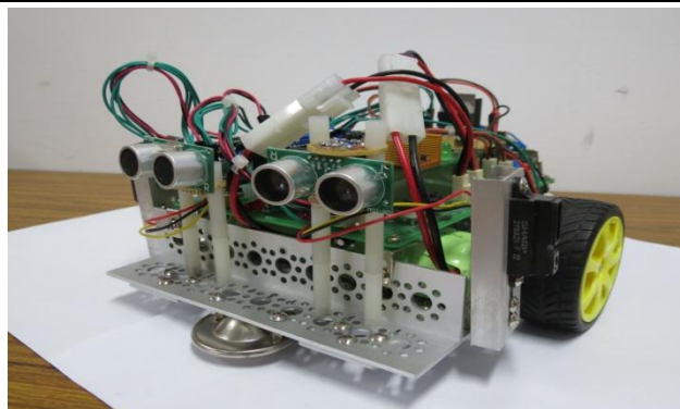
自走車背面
